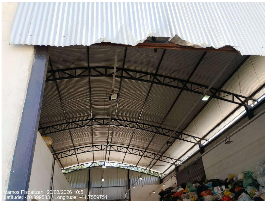
Cobertura e iluminação da área de triagem.
