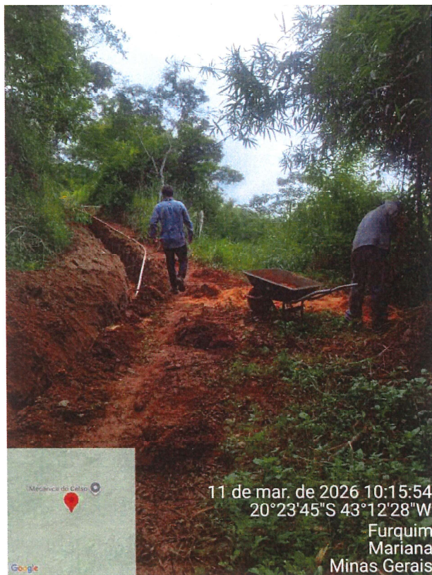
Fotos 3, 4, 5 e 6: Execução de serviço de instalação de rede adutora e de distribuição de água potável no Subdistrito de Margarida Viana
