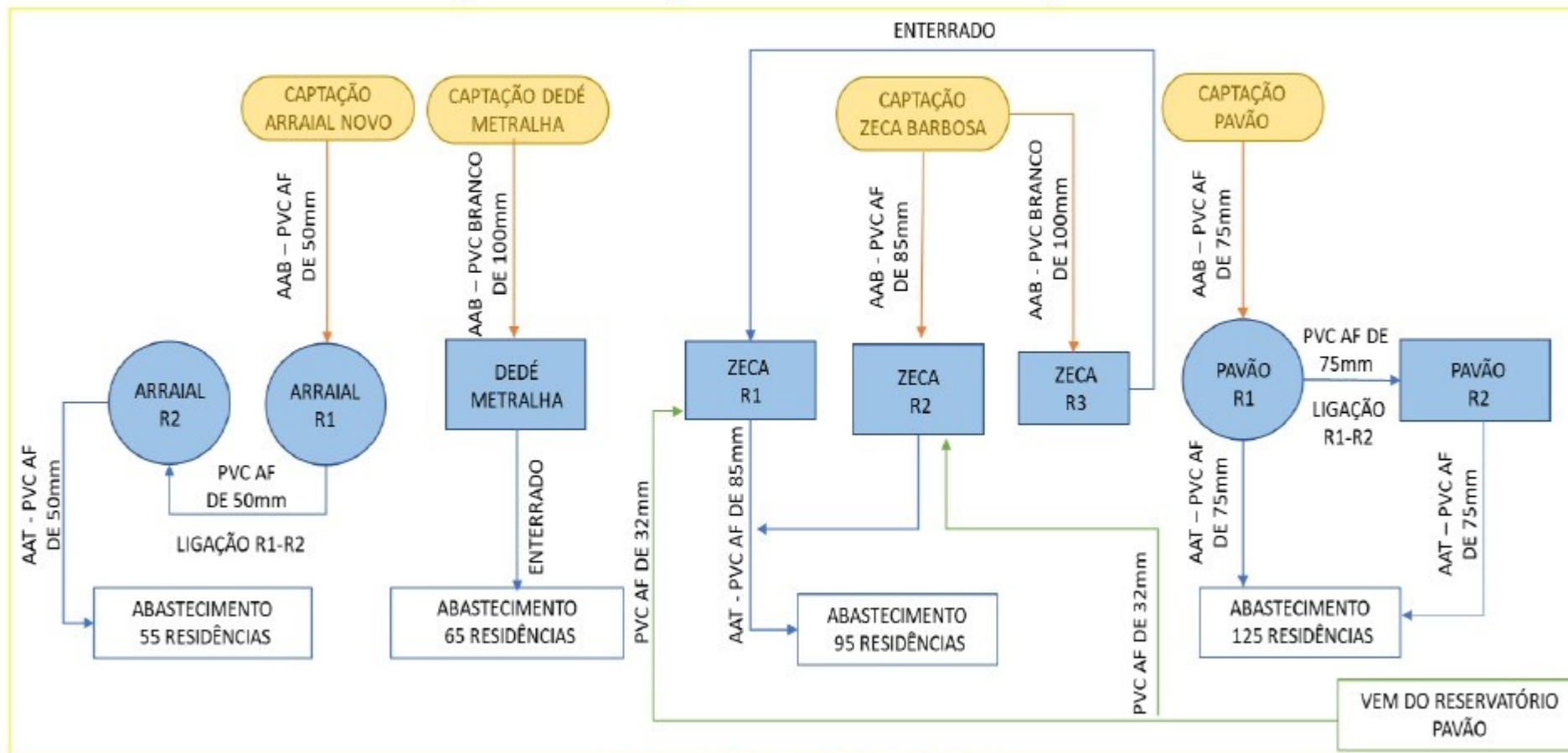
Figura 3 – Fluxograma Geral do SAA Furquim/MG
