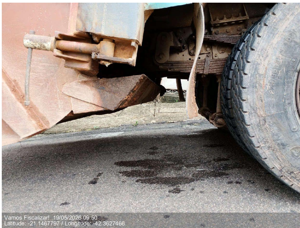
Vazamento na calha coletora de chorume.
